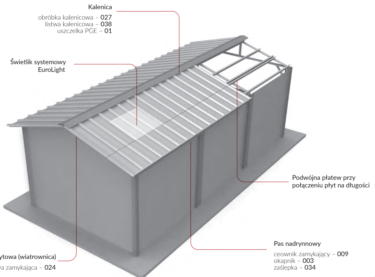
pojedynczy moduł
