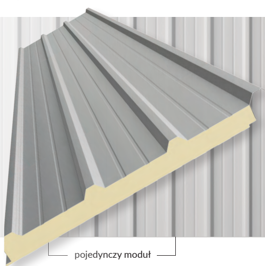
pojedynczy moduł
