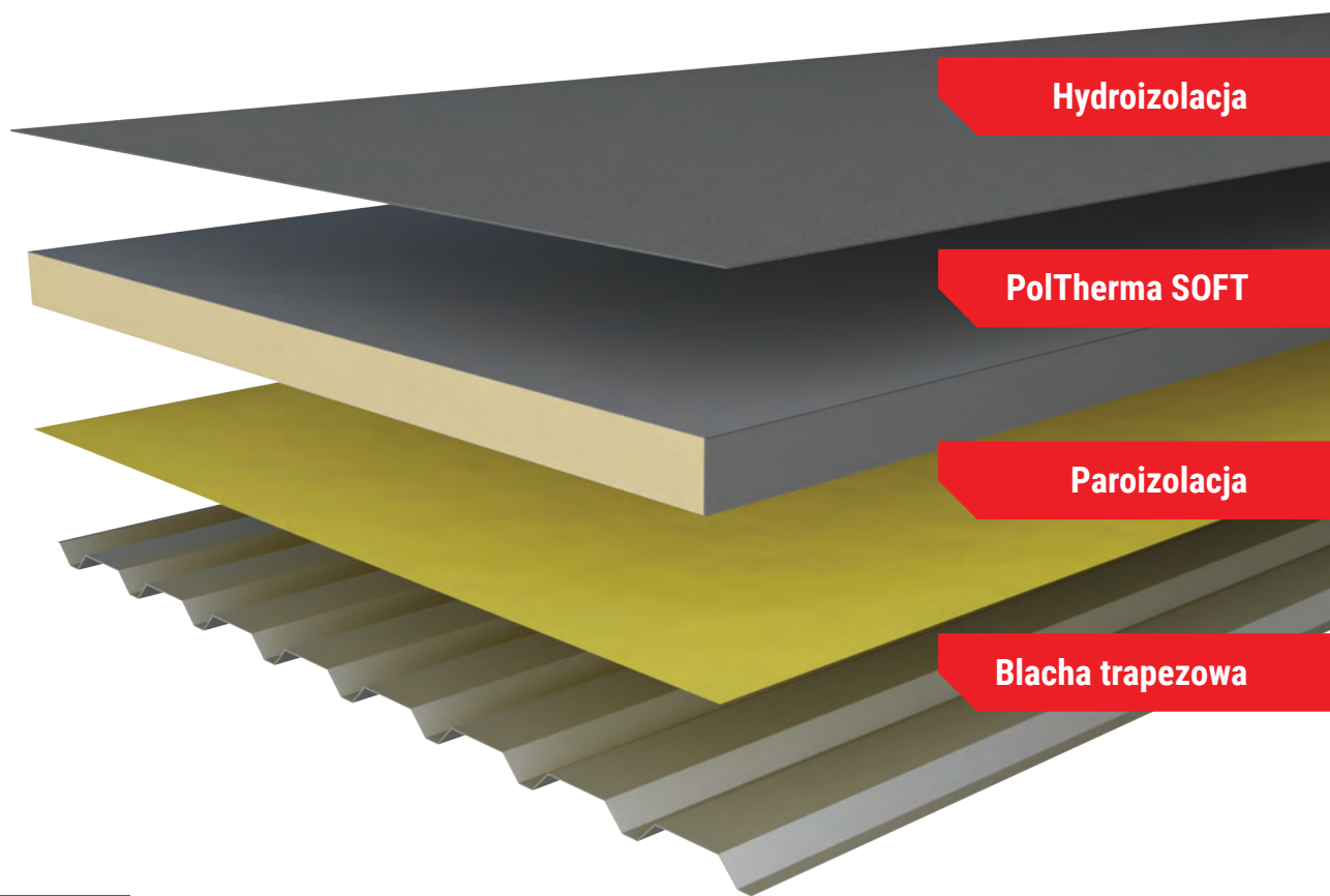
Przekrój płyt
