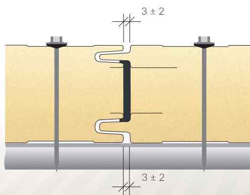
Przekrój styku płyt o grubościach 40 - 80mm:
