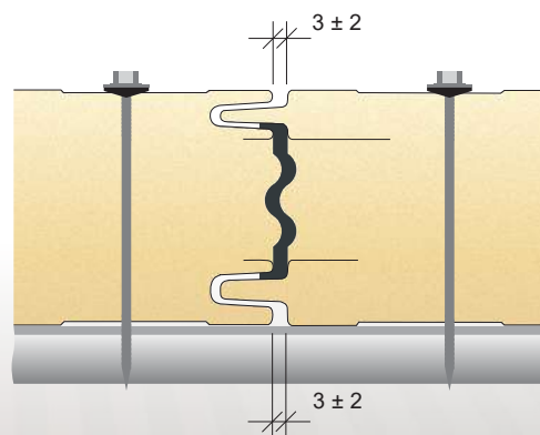
Przekrój styku płyt o grubościach 100 - 200mm:
