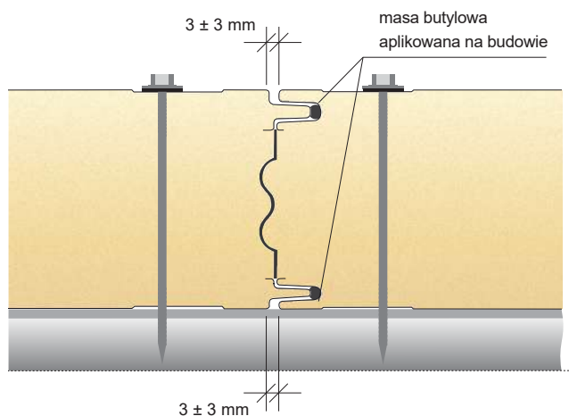
Przekrój styku płyt - styk zalewany
